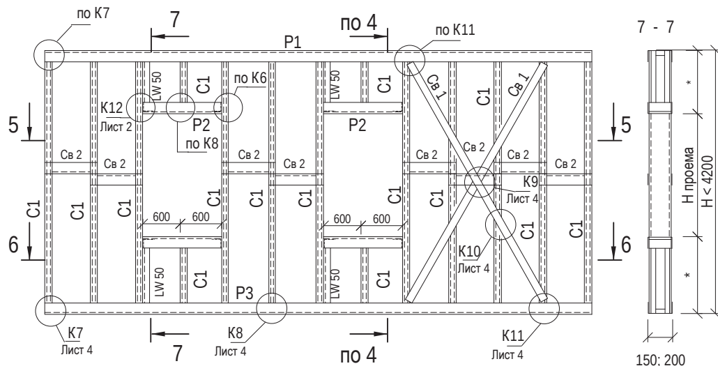
Фрагмент 2 каркаса с оконными проемами
