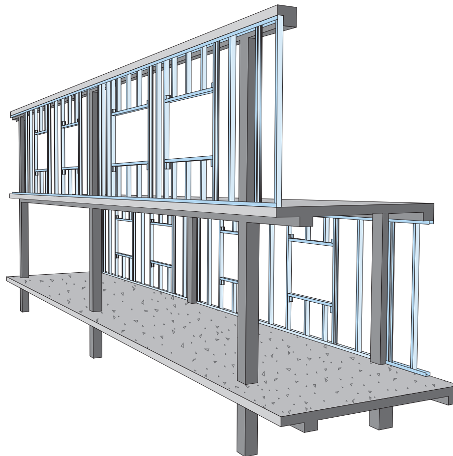
Рис. 1. Схематическое изображение здания со сборно-монолитным каркасом
