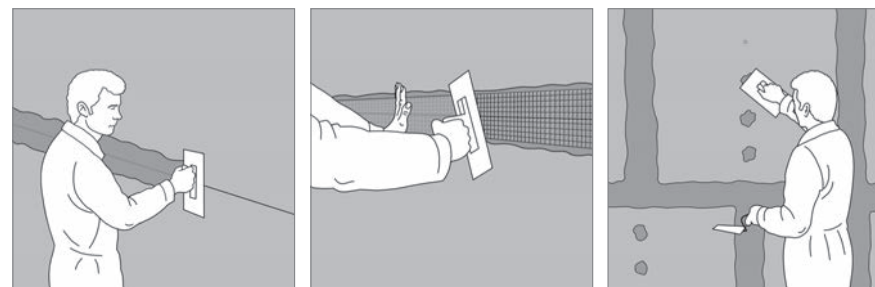
Рис. 15. Шпаклевание стыков и мест установки шурупов
