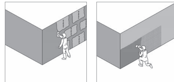
Рис. 22. Нанесение базового штукатурного слоя
