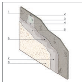
Рис. 17. Декоративное оштукатуривание наружной облицовки
