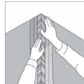
Рис. 20. Армирование углов
