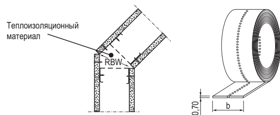
Рис 7. Соединение фрагментов каркаса стены под произвольным углом
